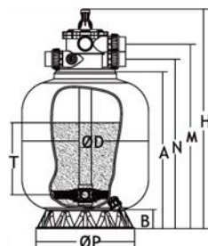
650-TM-2 ~ 1200-TM-2
